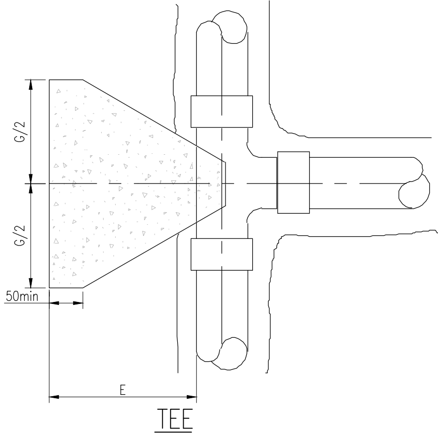
TEE
